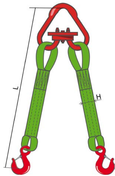
Двухветвевой
